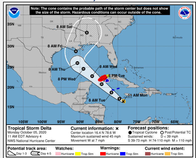
Pronóstico de trayectoria de TT Delta
