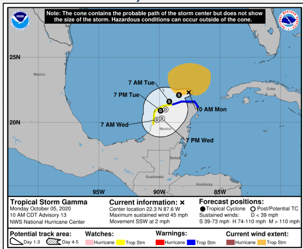
Pronóstico de trayectoria de TT Gamma
